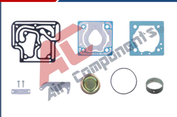
601.01.2300 REPUESTO MAYOR CON BUJE
