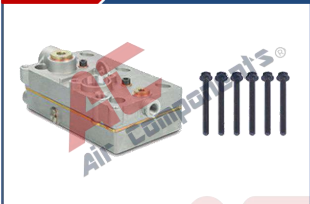
147.01.1200 CABEZA DE COMPRESOR
